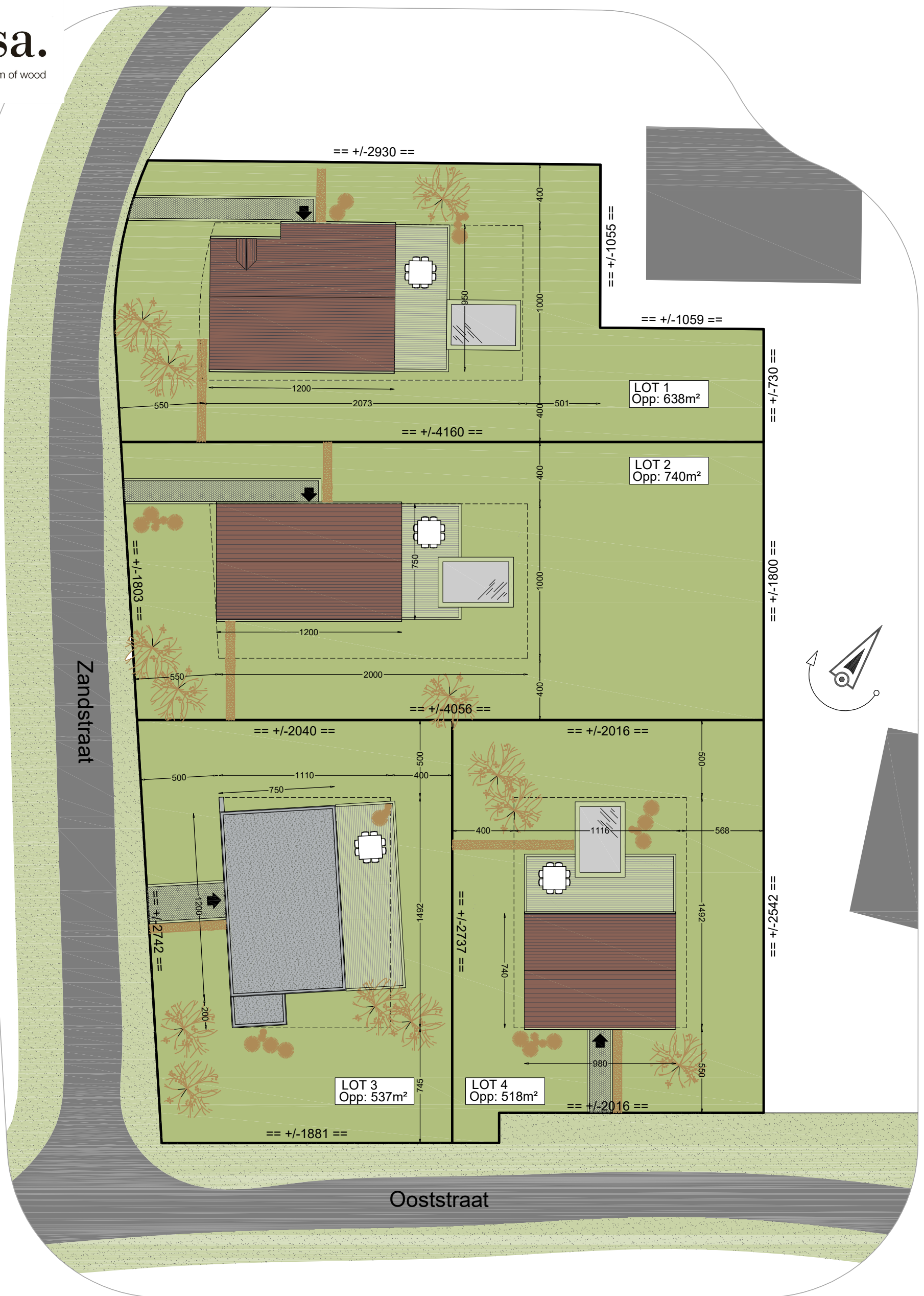
TERREINPLAN - schaal 1/200
